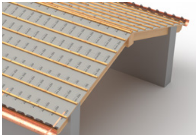
Singola orditura con listelli in legno
