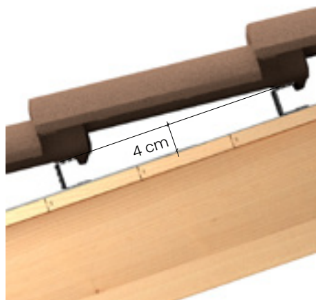
Interapedine con listello "UNO"
